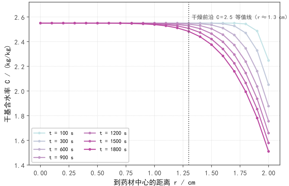
(b) 含水率场: 干燥完全限制在表层
