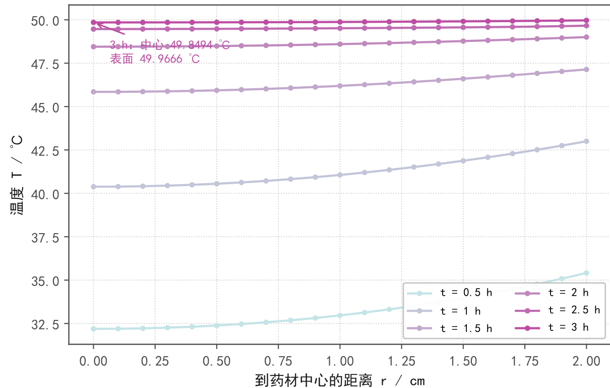
(a) 温度：3 h 内已接近烘房温度
