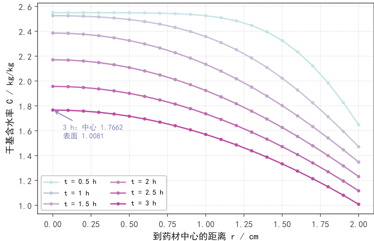
(b) 含水率：显著下降但远未达终点
