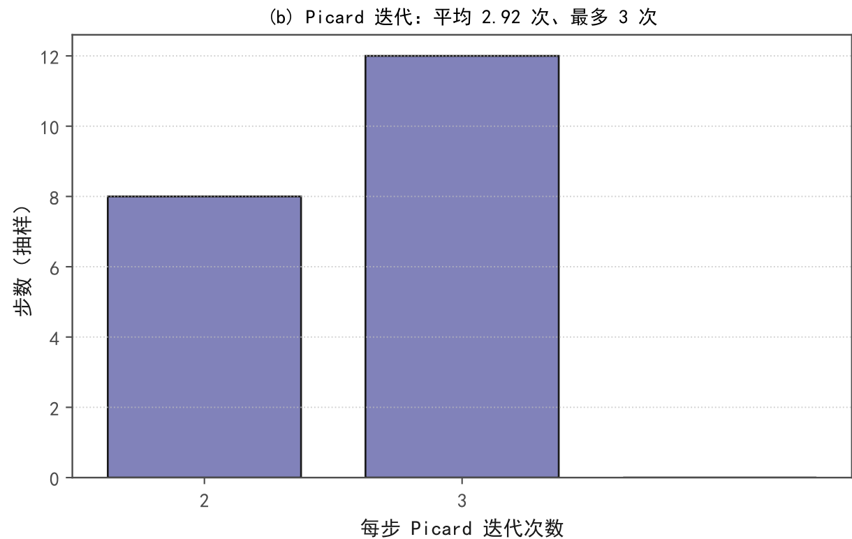
图 FIG-41 自适应时间步长与非线性迭代历史
