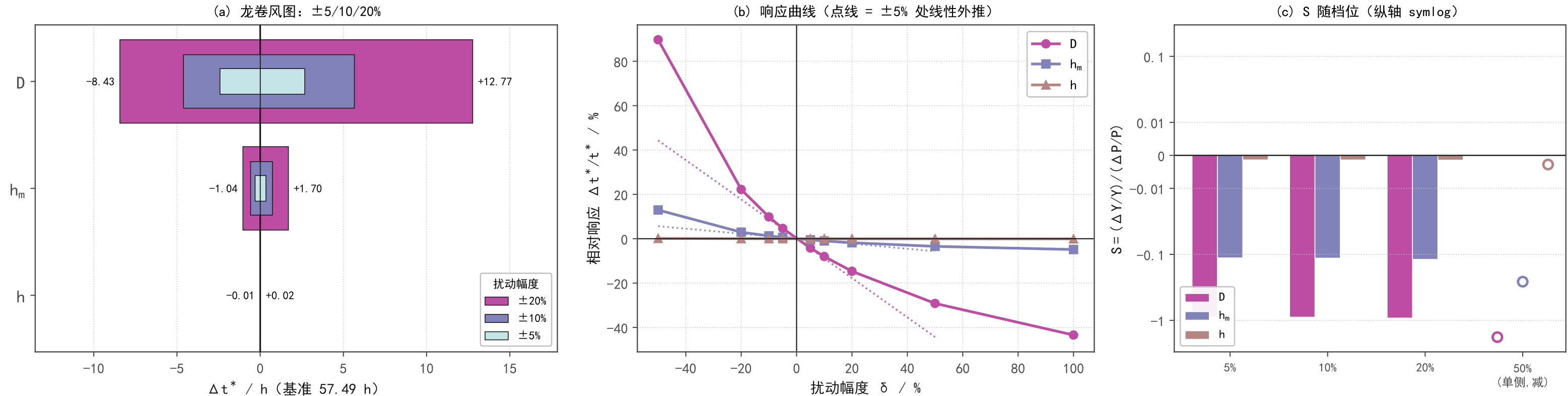
图 G13 参数灵敏度： |S_D| 在 \pm 5\% 处为 0.886、在 -50\% 处升至 1.794 —— 报「灵敏度系数」必须注明档位
