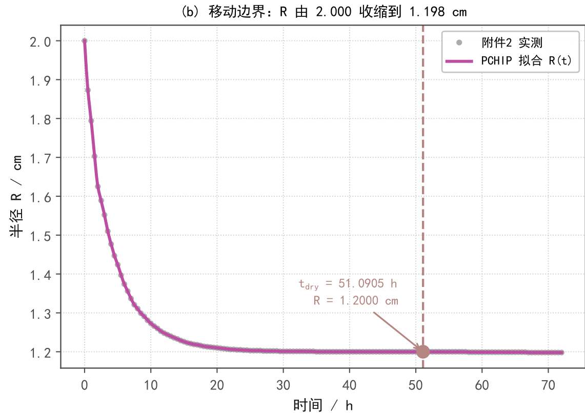
图 G7 问题4: 材料坐标下的收缩体干燥 ( \xi = r/R(t) , 无 \dot{R} 对流项)
