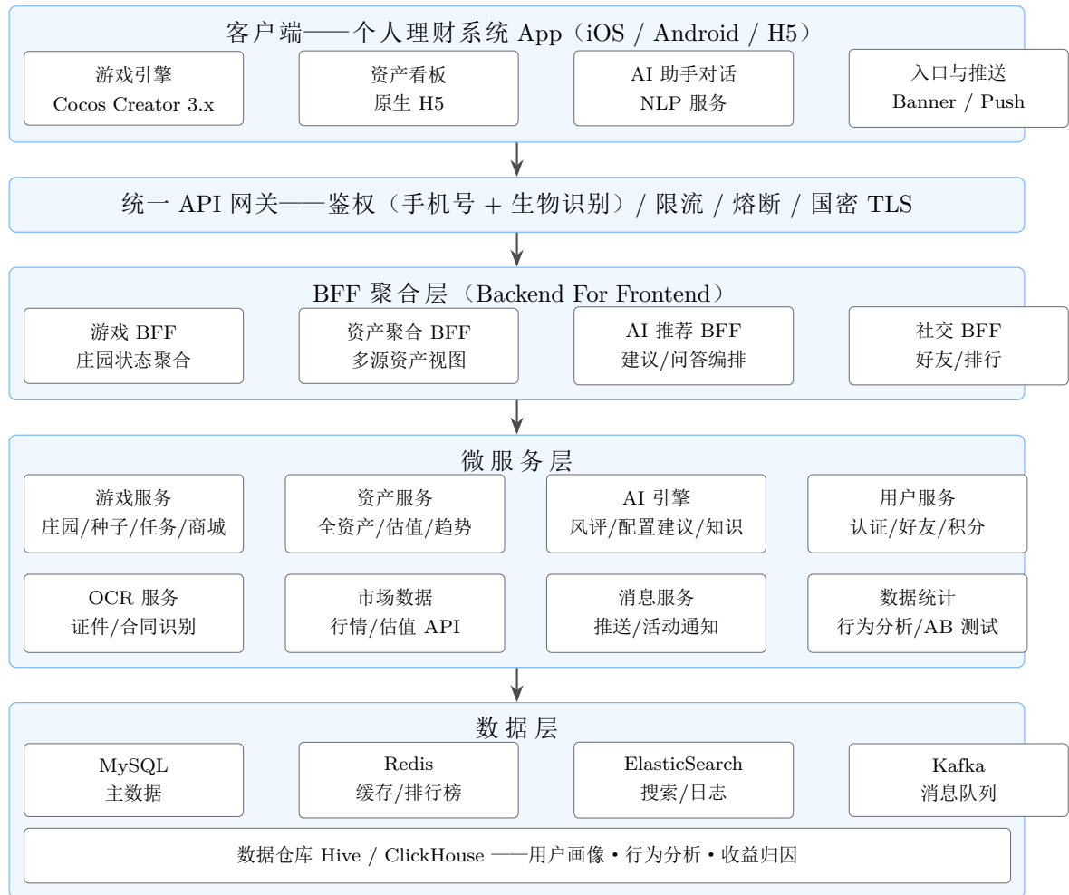
图 1: 财富庄园总体分层架构
