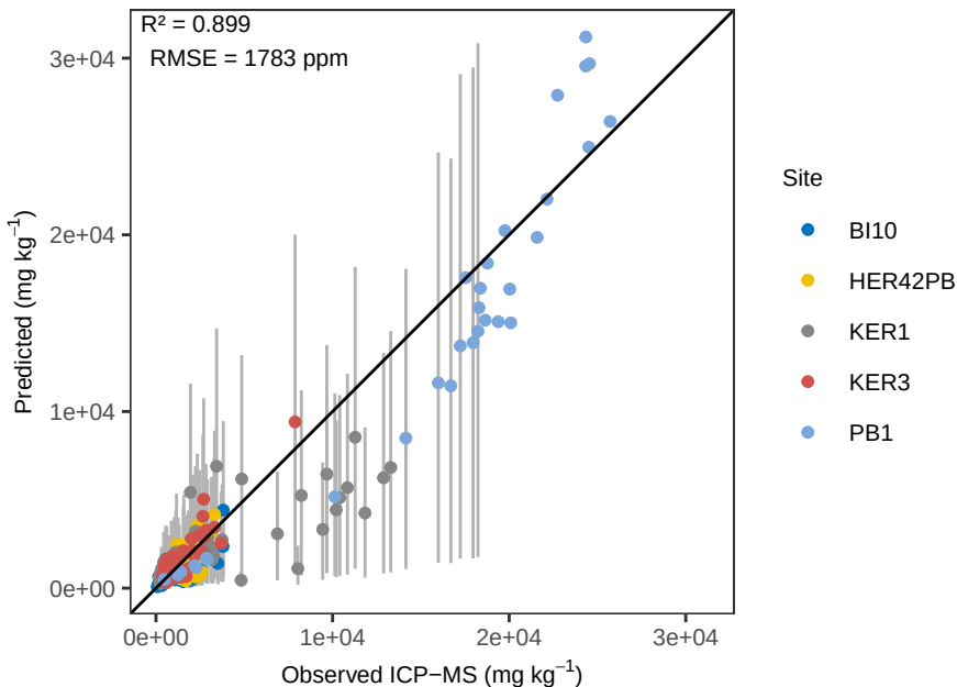
Ti Bayes – ACE Pred vs Ob (% err)
