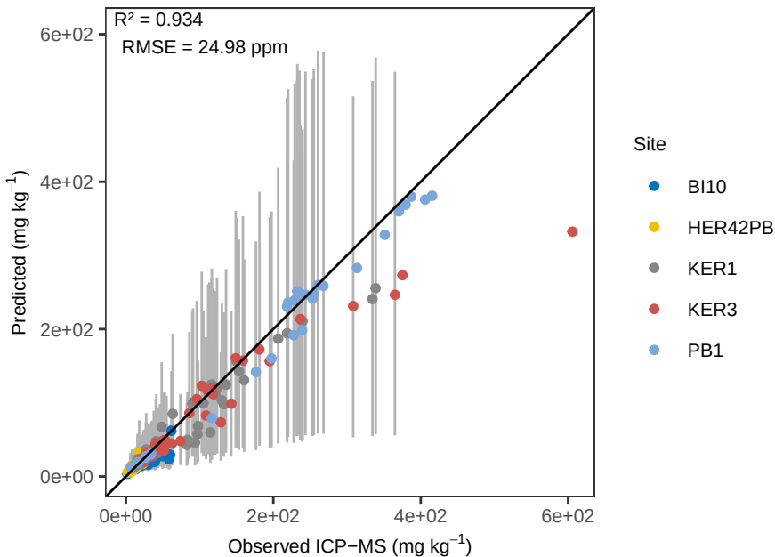
Zr RF – ACE Pred vs Ob (% err)
