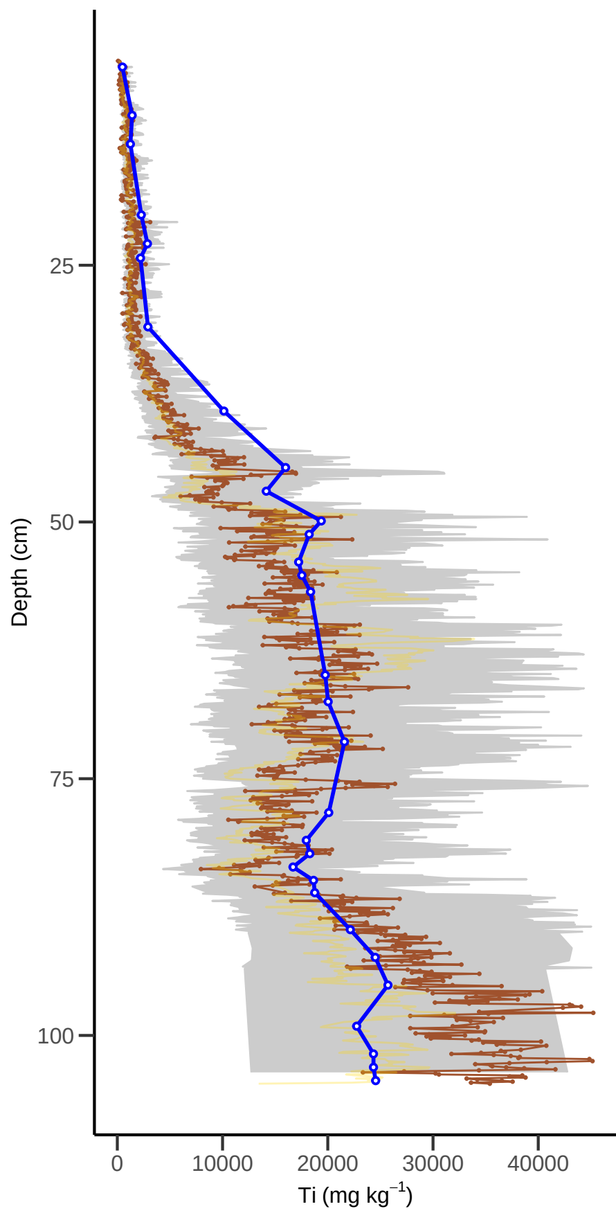
PB1 : PLS & WLS log_inc predicted vs ICP-MS
