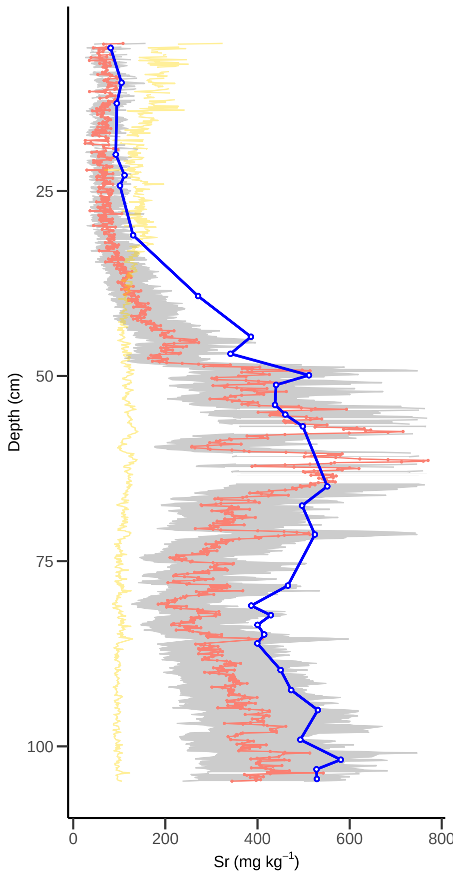
PB1 : PLS log_inc & clr predicted vs ICP-MS
