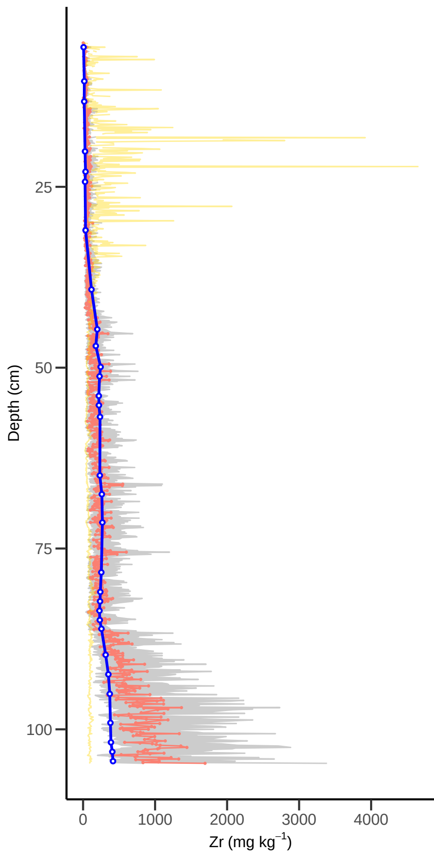
PB1 : PLS log_inc & clr predicted vs ICP-MS
