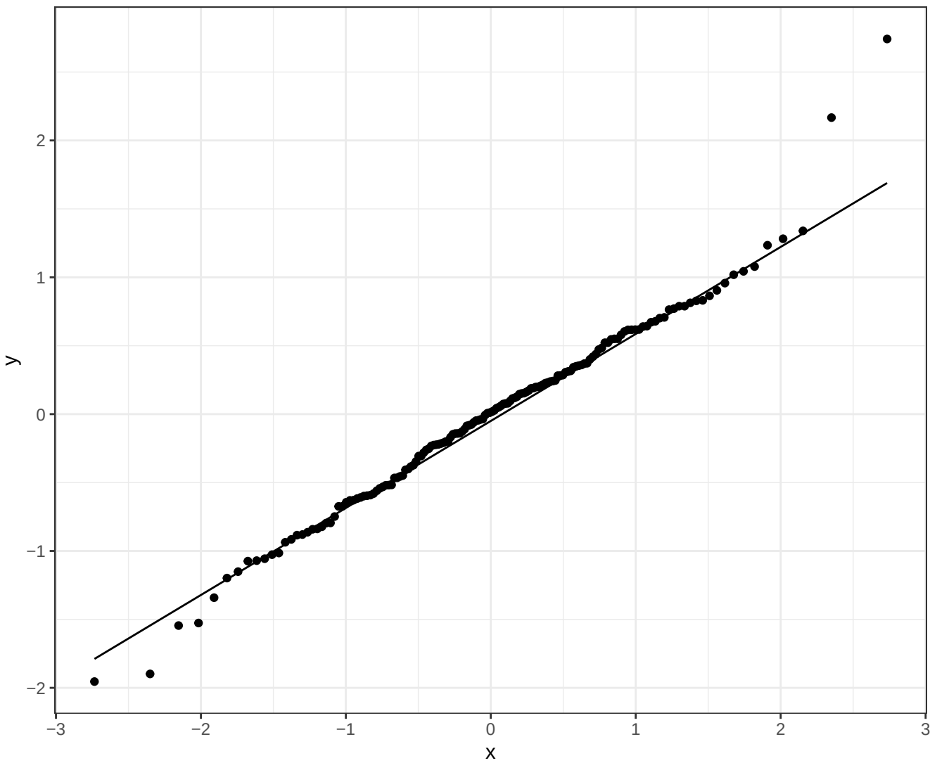
Ti Q-Q Plot
