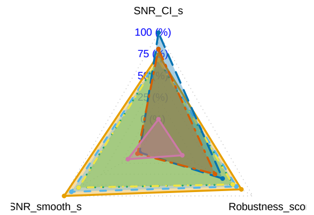
Ca - PB1
