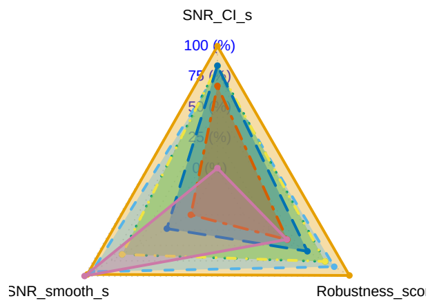
Ca - KER3
