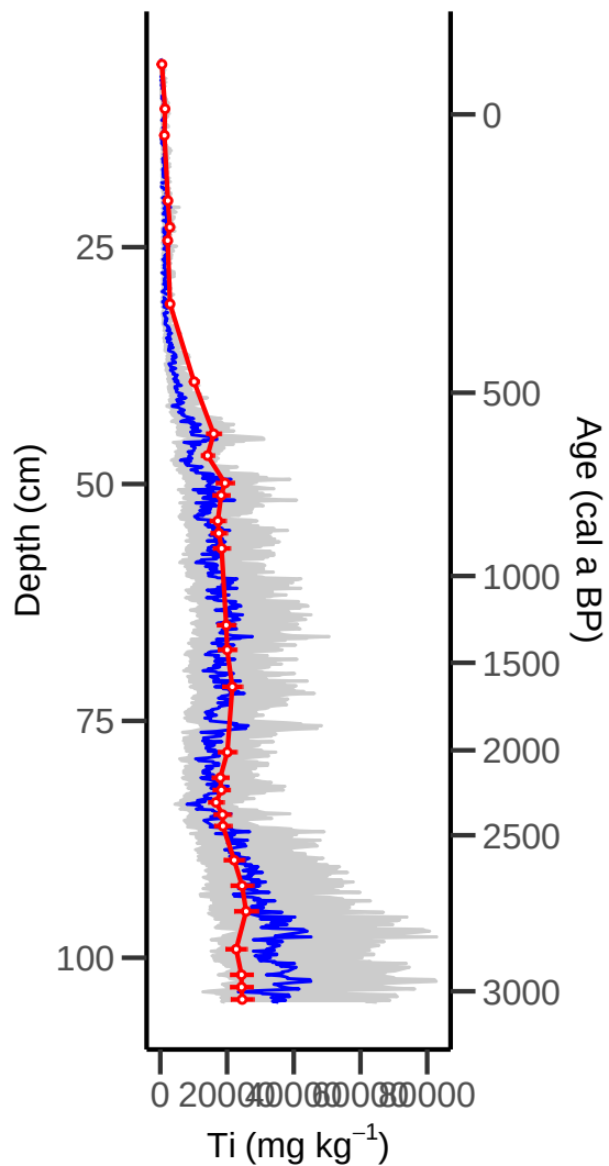
PB1: PLSR Ti Predictions wi
