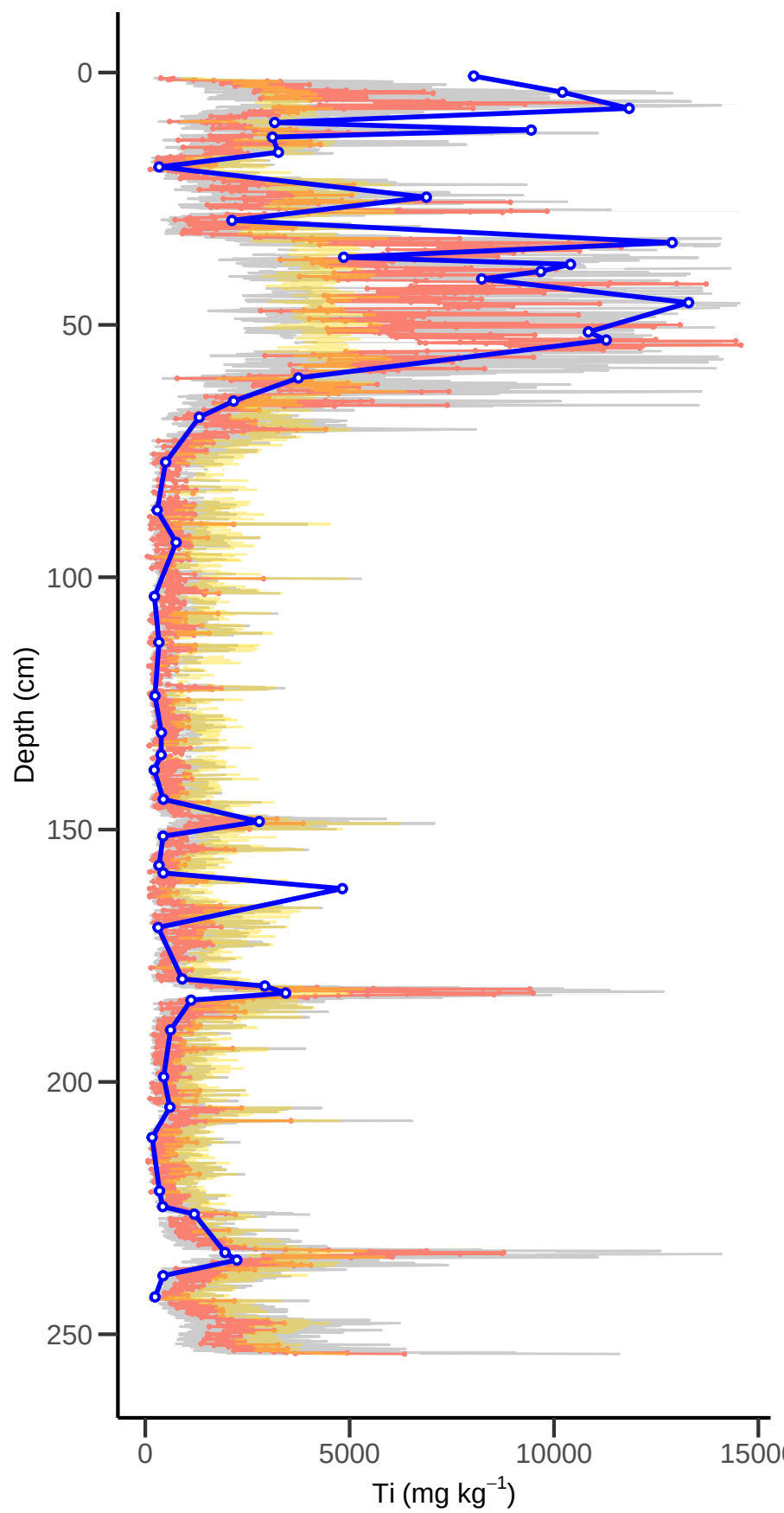
KER1 : PLS log_inc & clr predicted vs ICP-MS
