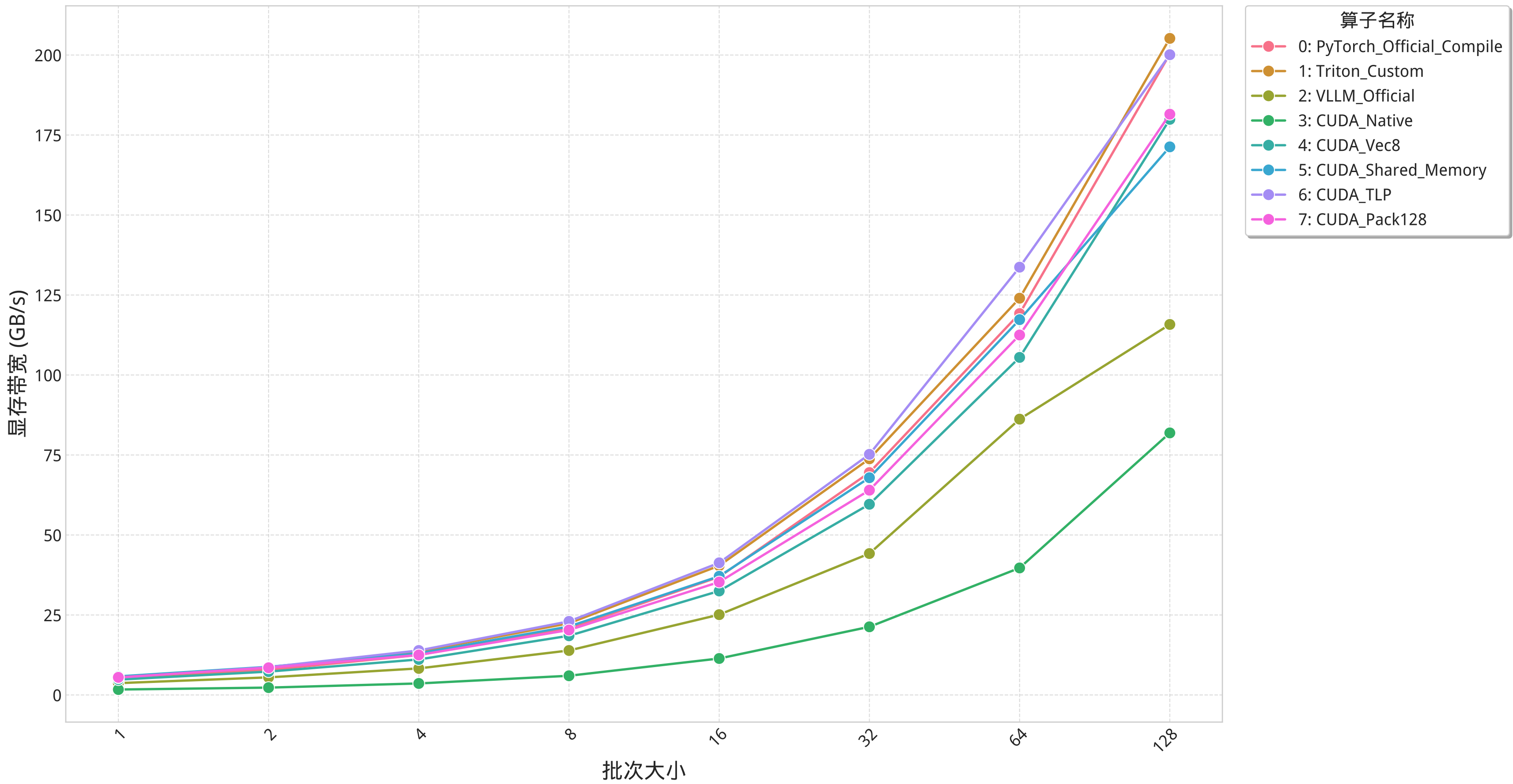
不同 RMSNorm 算子性能对比
