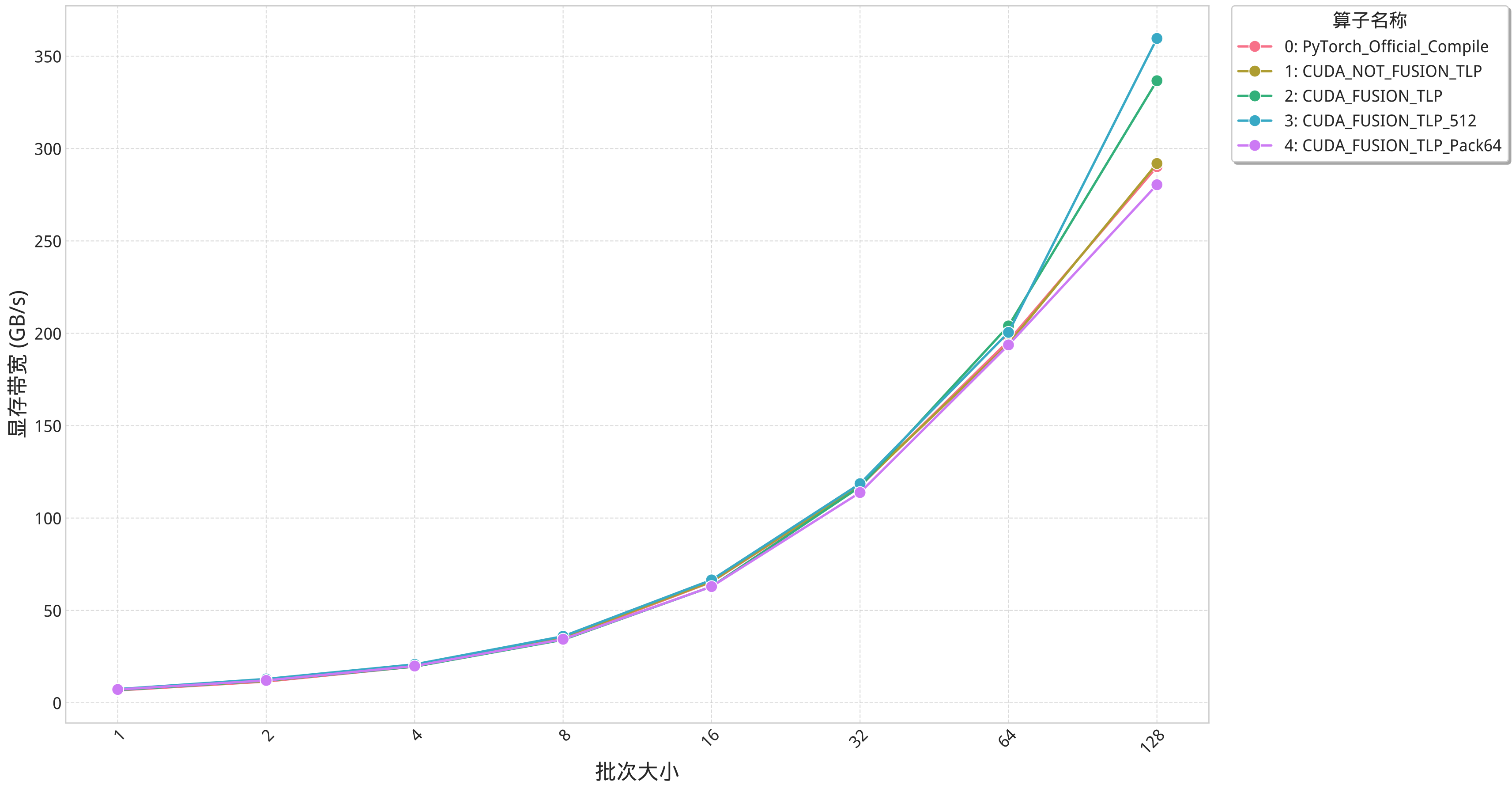
不同 Add-RMSNorm 算子性能对比
