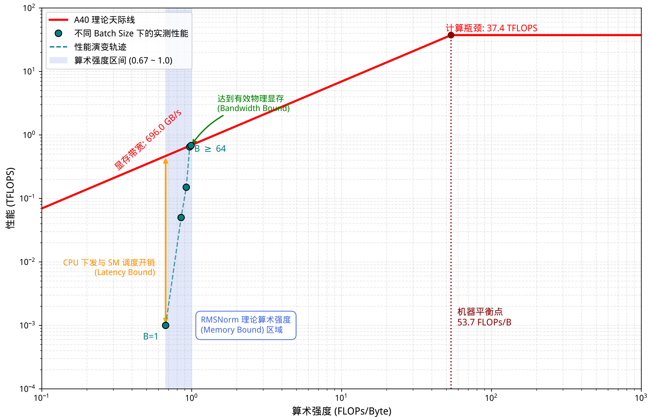
基于 NVIDIA A40 GPU 的 RMSNorm 算子 Roofline 性能分析
