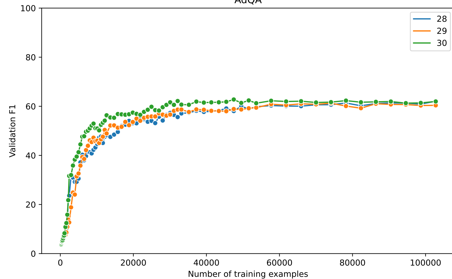
AdQA
