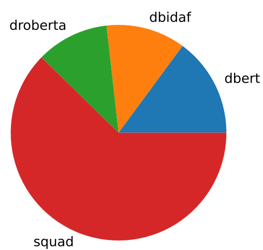
cluster 2 (n=1430)
