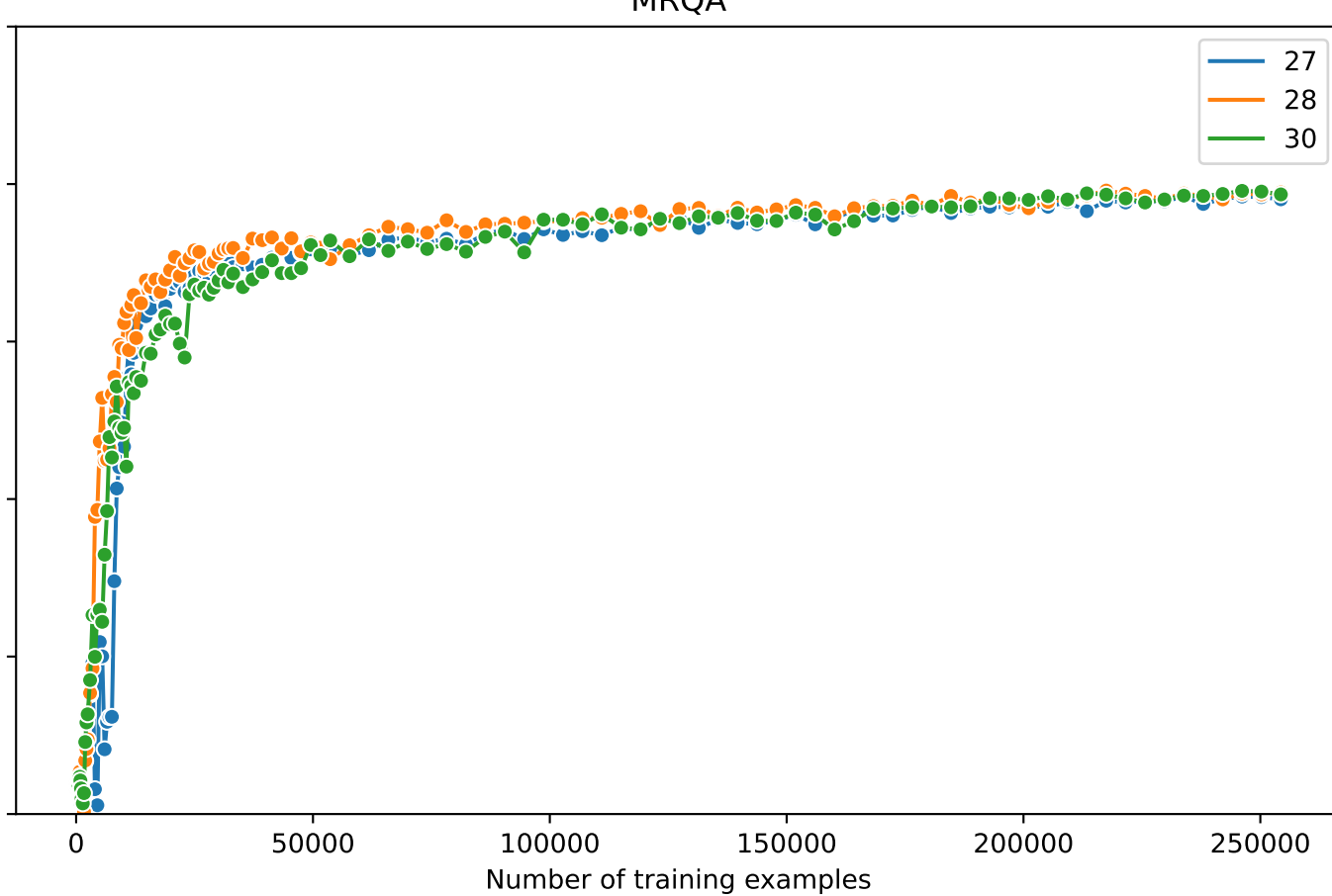
MRQA
