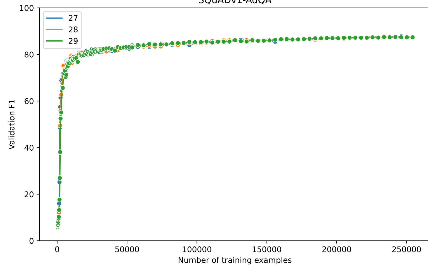
AdQA
