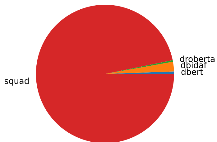
cluster 0 (n=7066)
