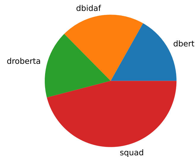
cluster 2 (n=446)
