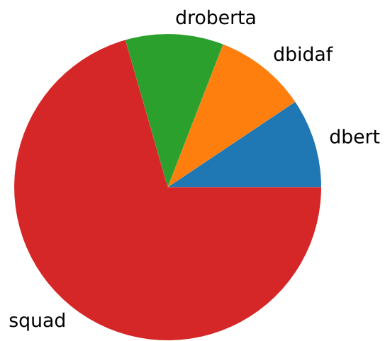
cluster 5 (n=2285)
