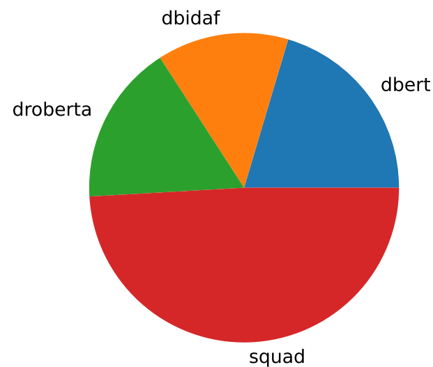
cluster 6 (n=1377)
