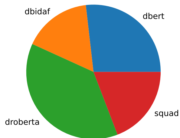
cluster 1 (n=824)
