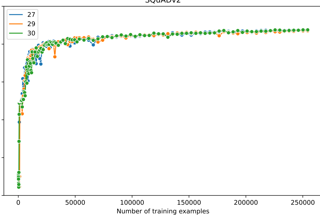
MRQA
