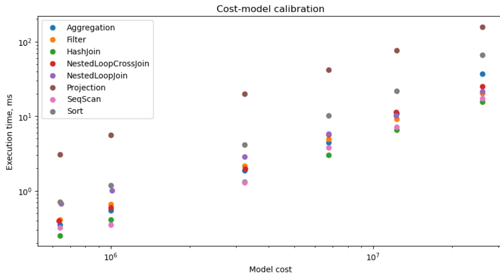
Рисунок 13 – Сопоставление расчетной стоимости физических операторов с фактическим временем выполнения.
