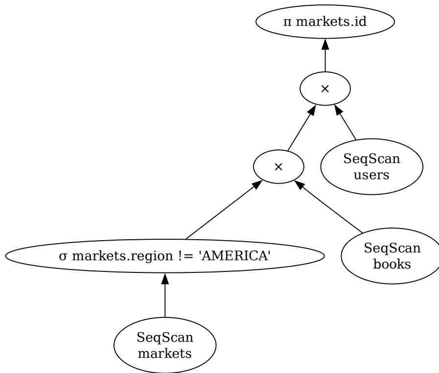
Рисунок 6 – Недостижимый физический план Microsoft SQL Server после конвертации для запроса из листинга 16
