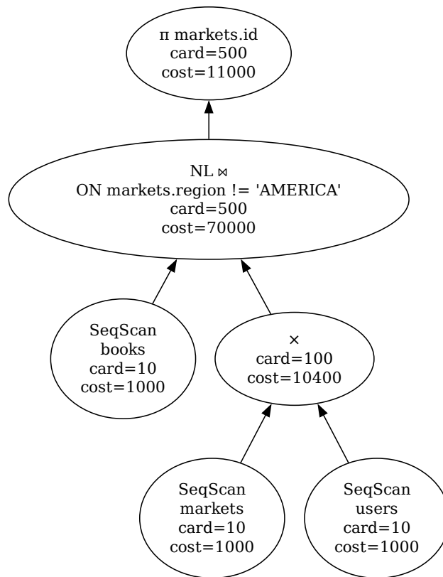
Рисунок 7 – Физический план, построенный модельной СУБД для запроса из листинга 16.
