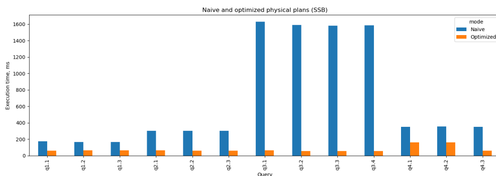
Рисунок 8 – Сравнение времени выполнения запросов при наивном и оптимизированном построении физического плана.
