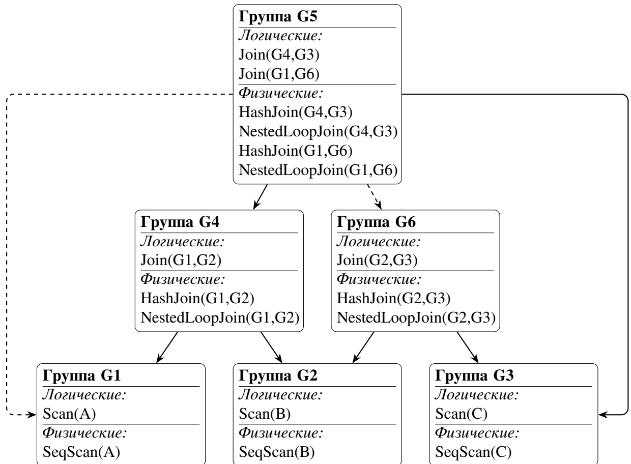
Рисунок 12 – Пример структуры Мемо.
