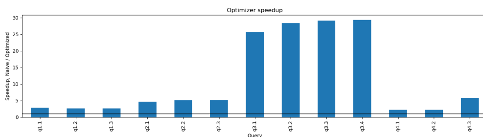
Рисунок 9 – Относительное ускорение выполнения запросов после применения оптимизатора.
