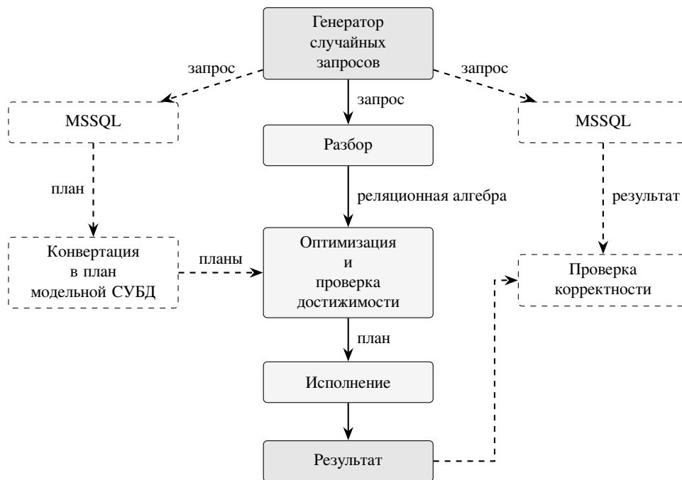
Рисунок 5 – Процесс обработки запроса в модельной СУБД.
