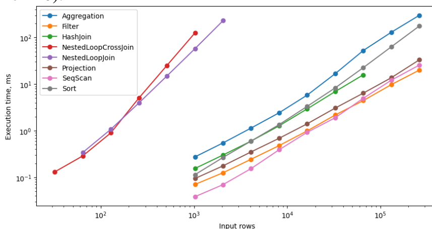
Рисунок 10 — Зависимость времени выполнения физических операторов от размера входных данных.
