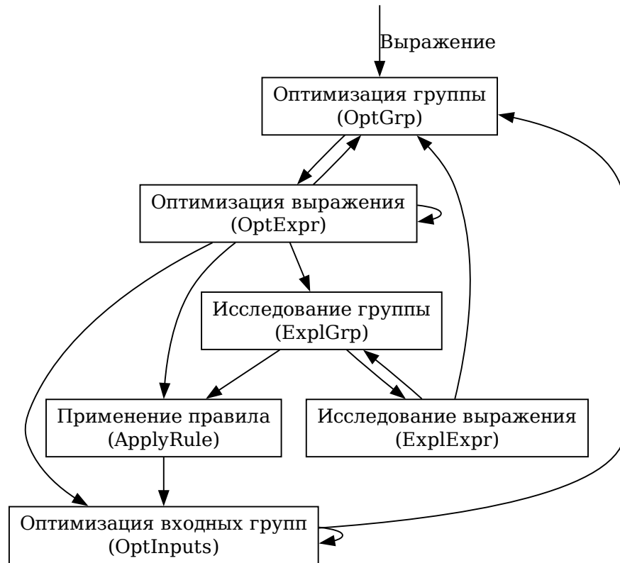
Рисунок 11 – Схема взаимодействия задач в оптимизаторе Cascades
