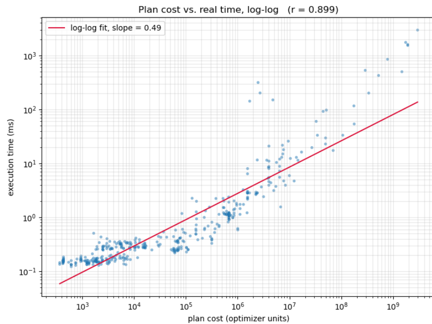
Рисунок 15 – Сравнение скорости выполнения и стоимости на случайных запросах.
