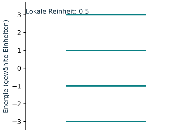
Verschränkter Grundzustand
