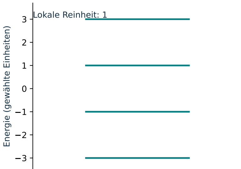
Produkt-Grundzustand
