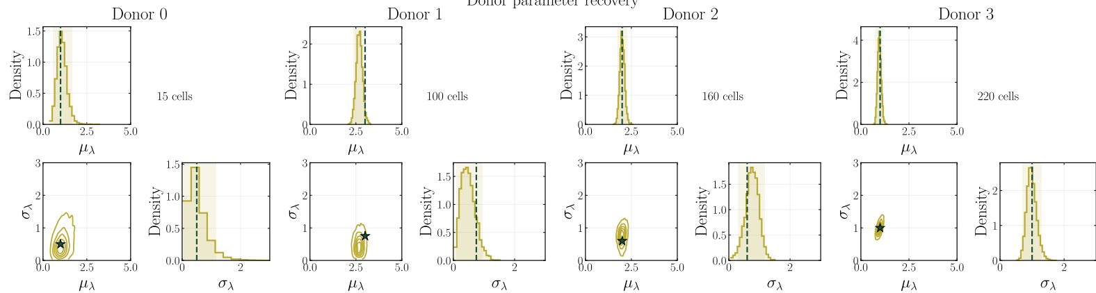
Donor parameter recovery
