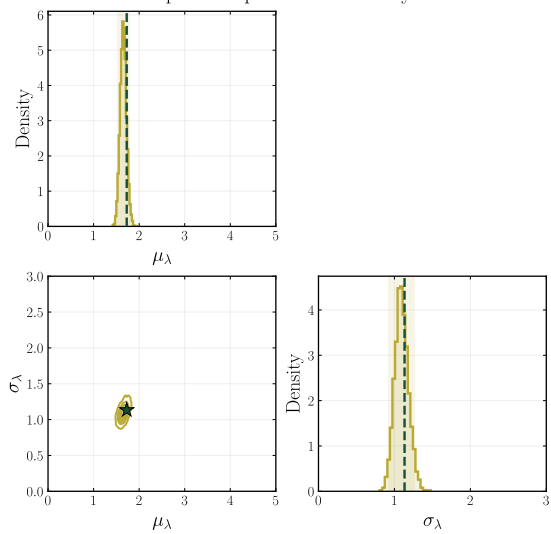
Population parameter recovery
