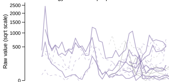
Mesocentrotus franciscanus – Biomass
