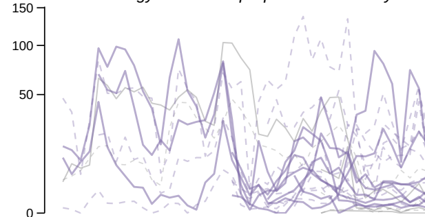
Mesocentrotus franciscanus – Density
