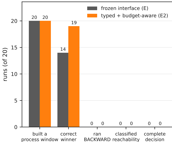
a decision chain, mini at 175 CU
