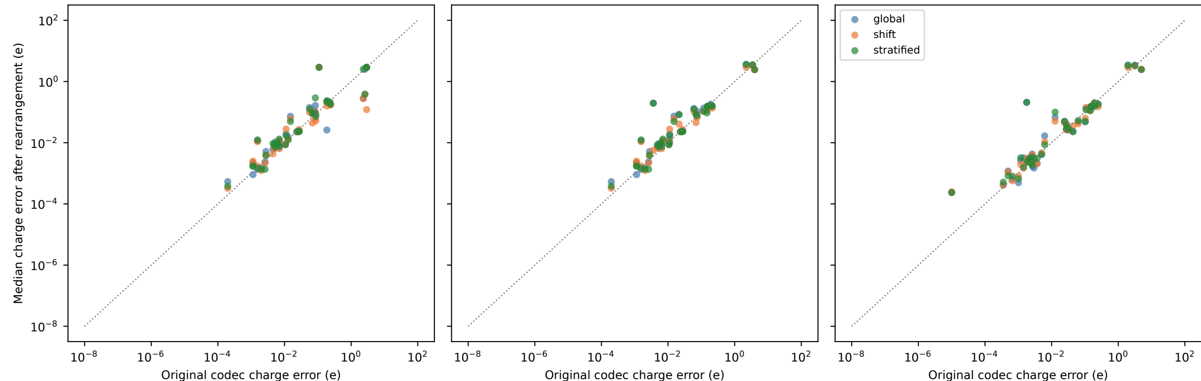
BaderKit ongrid
