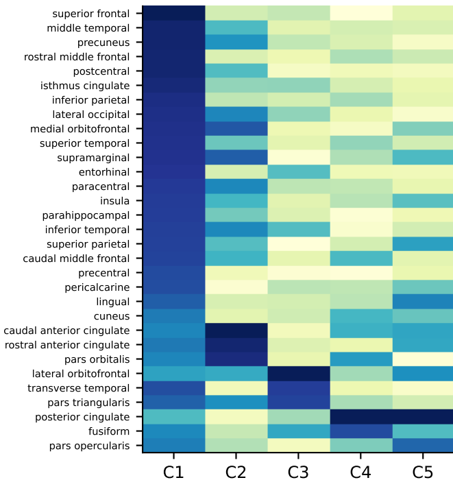
PCA loadings
