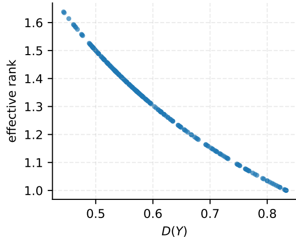
(c) D = 1/ER - 1/k
