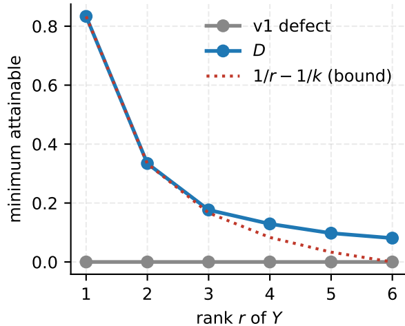
(b) rank-deficient matrices
