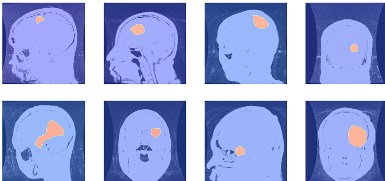
(a) Actual
