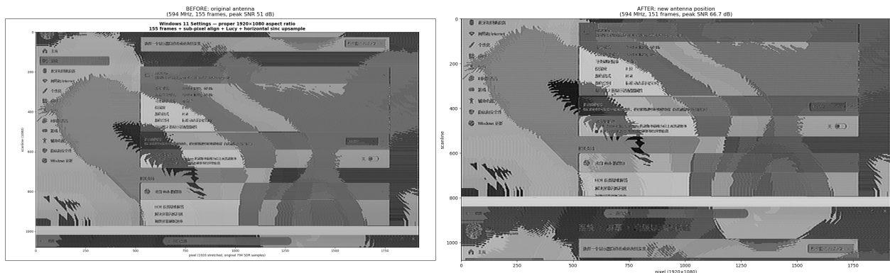
Figure 2: 天线位置调整前后重建对比 (同一 Win11 Settings 画面，同 594 MHz 谐波)。左：原始位置；右：方向 + 距离微调后，峰值 SNR +16 dB，HSYNC SNR > 4 \times 。Phase 1 W2 阶段优先做天线参数化扫描可在零器件投入下取得最大 SNR 改善。
