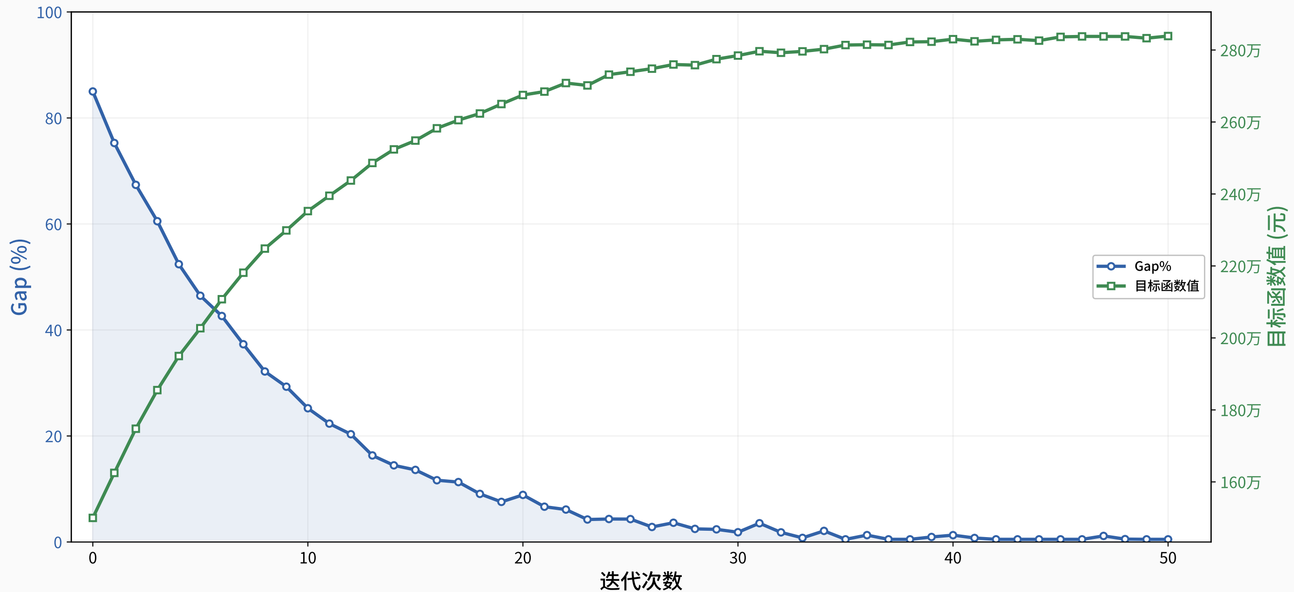
算法收敛过程 — Gap与目标函数值双轴对比
