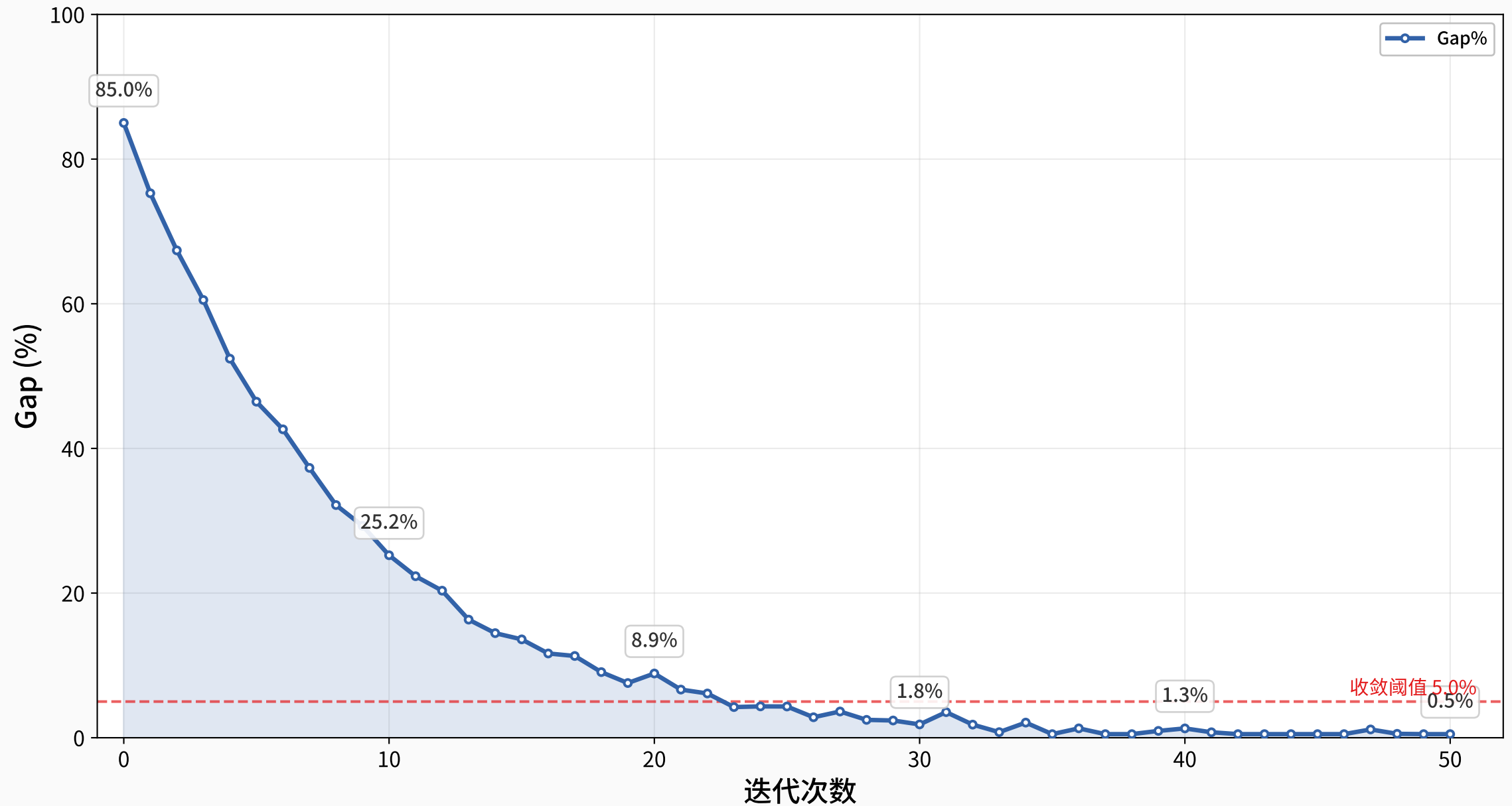
算法收敛曲线 — Gap随迭代次数变化
