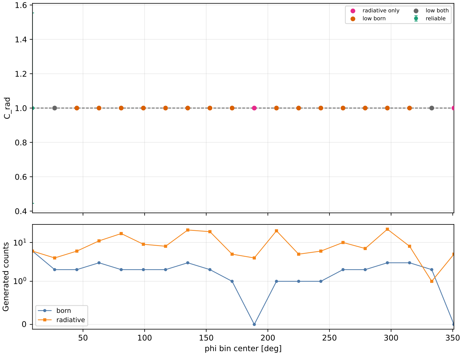
Radiative correction vs phi Q2 1.5-2, xB 0.1-0.15, -t 1.5-2
