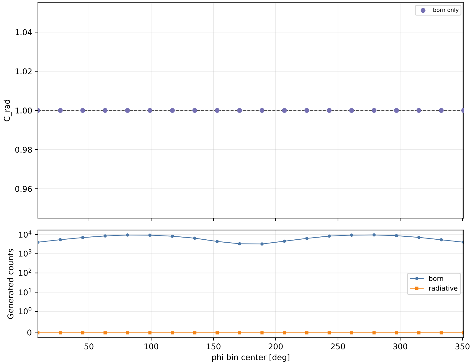
Radiative correction vs phi Q2 1.5-2, xB 0.58-0.7, -t 1.5-2
