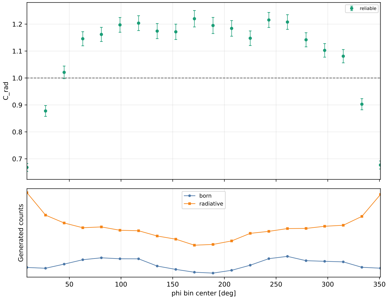
Radiative correction vs phi Q2 1.5-2, xB 0.25-0.3, -t 1.5-2
