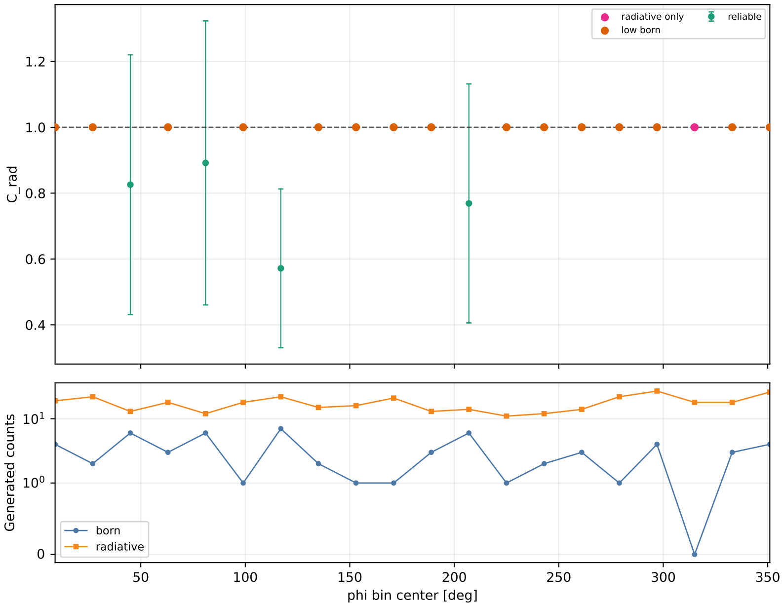
Radiative correction vs phi Q2 1.5-2, xB 0.1-0.15, -t 1.5-2
