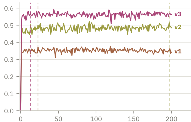
HitRate@10
