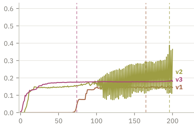
HitRate@10
