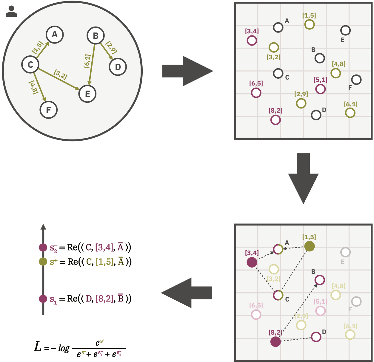
Σχήμα 4.11: Συνολική αρχιτεκτονική της τελικής υλοποίησης (v3), από τον γράφο του χρήστη έως την απώλεια. Ο CompGCN encoder παράγει embeddings των κόμβων και των τύπων ακμών (πάνω), από τα οποία συναρμολογείται μια τριπλέτα (h, r, t) (κάτω δεξιά). Στην συνέχεια ο ComplEx decoder μετατρέπει κάθε τριπλέτα σε ένα βαθμωτό score s = \text{Re}(\langle h, r, \bar{t} \rangle) (κάτω αριστερά). Η InfoNCE συγκρίνει το score της θετικής ακμής με εκείνα K αρνητικών, και το gradient της αναμορφώνει τα embeddings.
