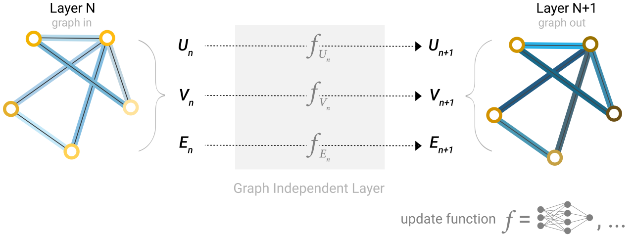
Σχήμα 2.9: Ένα GNN layer: Τα χαρακτηριστικά του γράφου διέρχονται από ένα MLP (βλ. Εν. 2.1.2) και παράγουν έναν ανανεωμένο γράφο [24].
