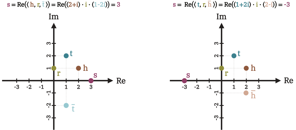
Σχήμα 4.7: Το ComplEx decoder βαθμολογεί μια τριπλέτα (h, r, t) , όπου h (head) = trigger device, r (relation) = rule, t (tail) = action device, με το τριγωναμικό γινόμενο \text{Re}(\langle h, r, \bar{t} \rangle) στο μιγαδικό επίπεδο, όπου \bar{t} το συζυγές του tail. Επειδή η εναλλαγή των ρόλων head/tail μετακινεί την συζυγία, το score που ανατίθεται στον κανόνα « h \rightarrow t » s = \text{Re}(\langle h, r, \bar{t} \rangle) (αριστερά) είναι διαφορετικό από αυτό που ανατίθεται στον κανόνα « t \rightarrow h » s = \text{Re}(\langle t, r, \bar{h} \rangle) . Αυτή η ιδιότητα επιτρέπει την αναπαράσταση κατευθυνόμενων κανόνων.
