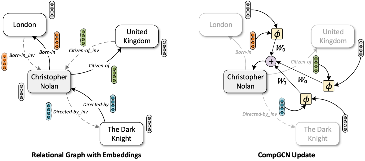
Σχήμα 4.6: Η αρχιτεκτονική του CompGCN: κάθε μήνυμα συνθέτει την αναπαράσταση του γείτονα με εκείνη του τύπου της ακμής που τους συνδέει μέσω της συνάρτησης σύνθεσης \phi [50].
