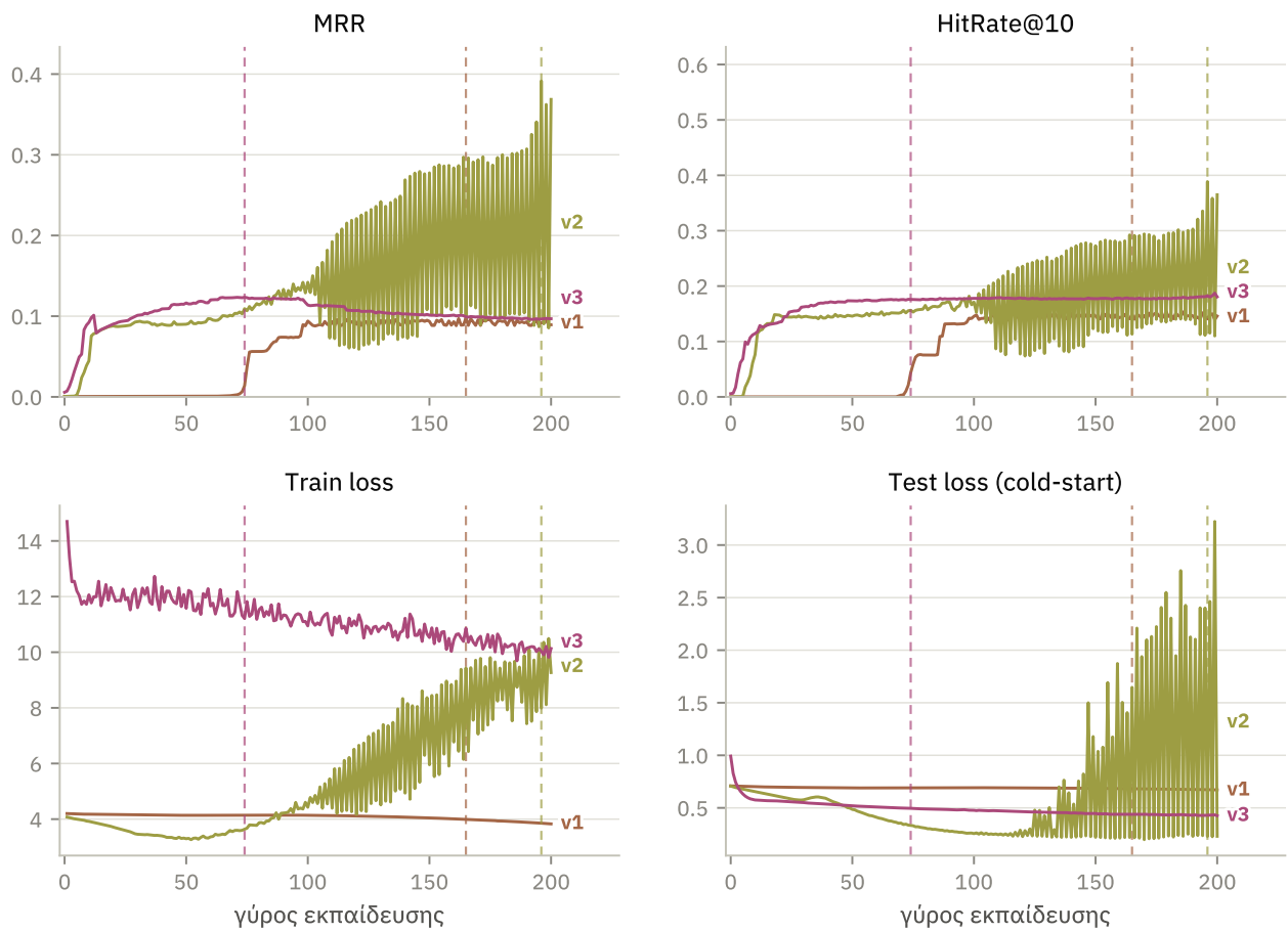
Σχήμα 5.7: Σύγκριση των τριών εκδόσεων στο σενάριο true cross-device. Είναι εμφανής η έντονη αστάθεια των καμπυλών, ιδιαίτερα της v2.
