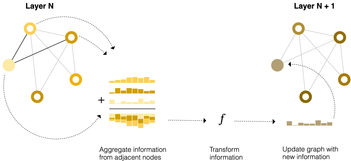
Σχήμα 2.10: Η διαδικασία του message passing: ο κόμβος με γέμισμα (αριστερά) κάνει aggregate πληροφορία από τον εαυτό του και τους δύο γείτονές του και ανανεώνει την κατάστασή του (δεξιά) μέσω μιας update function. Η διαδικασία γίνεται σε κάθε κόμβο του γράφου [24].
