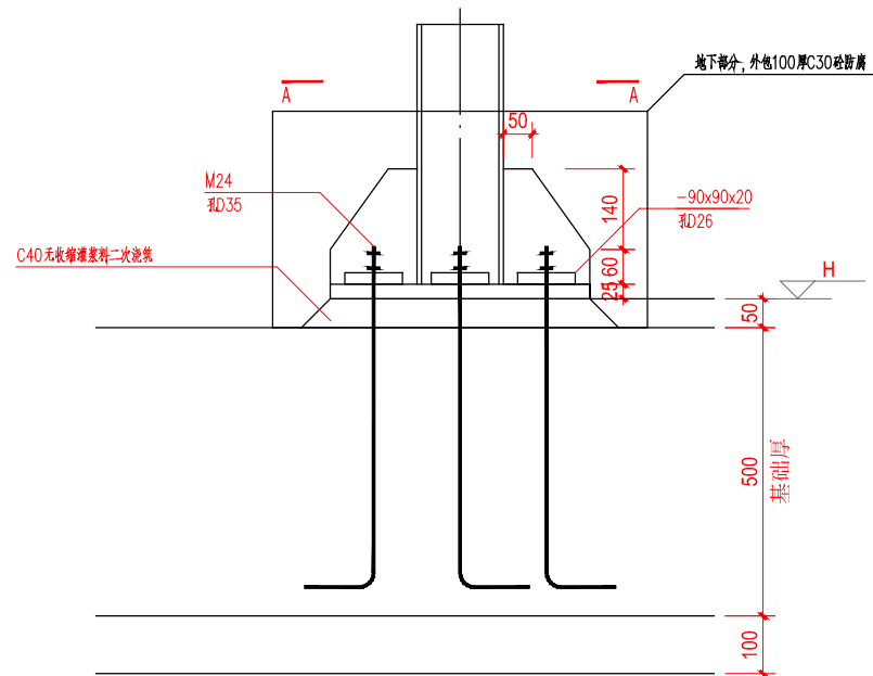
钢柱脚节点 1:10
