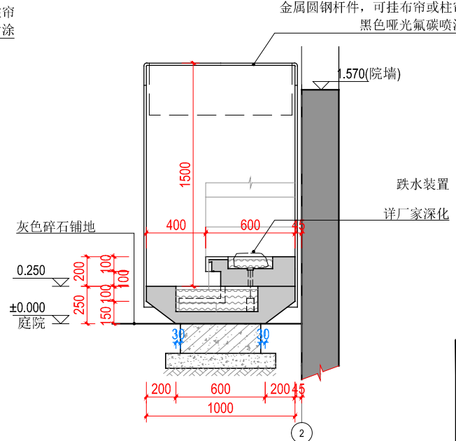
11 剖面大样图 1:20
