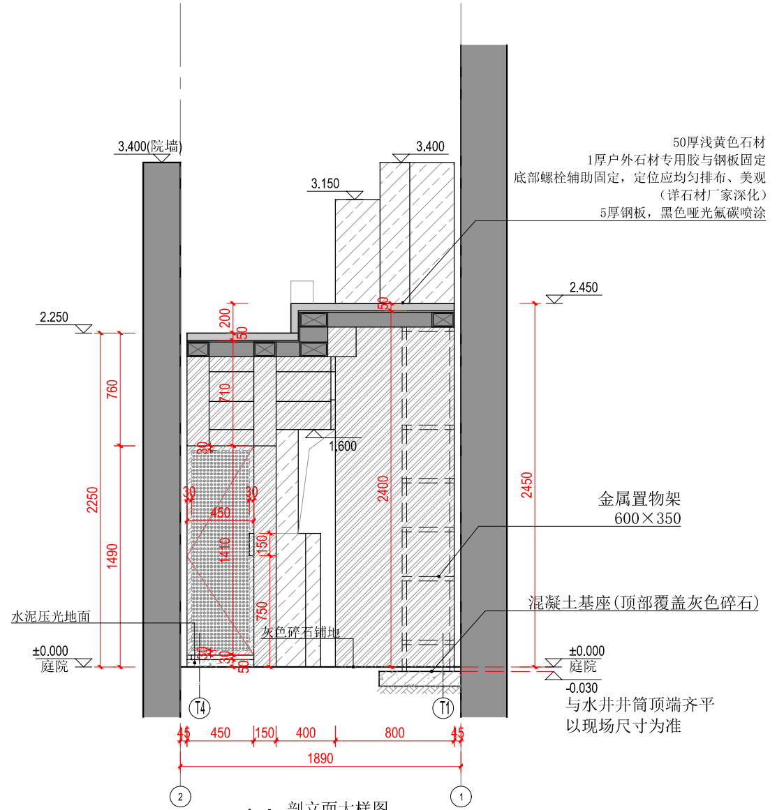
14 剖面大样图 1:20
