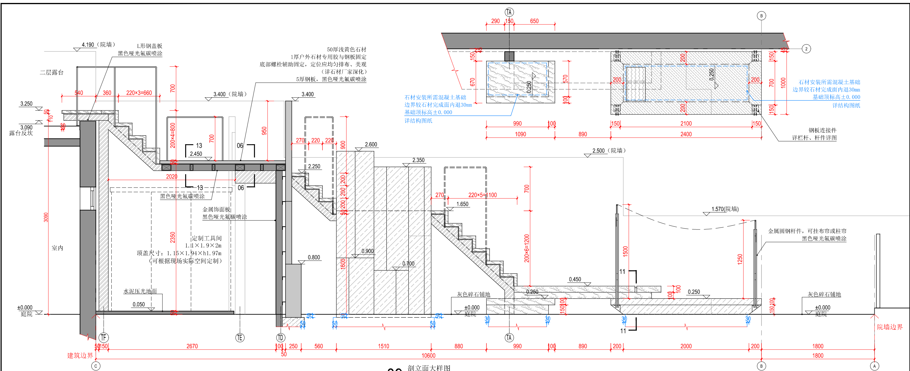
09 剖面大样图 1:20
