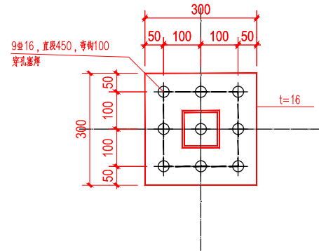
幕墙柱脚埋件
