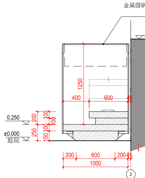
10 剖面大样图 1:20
