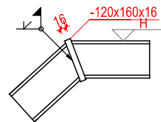
梯梁转折节点 1:10
