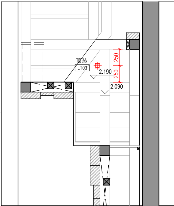
局部天花灯具定位尺寸图
