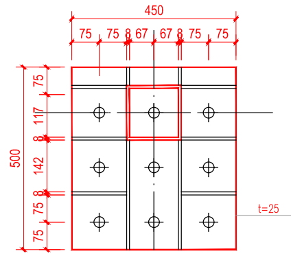
A-A 偏心柱脚
