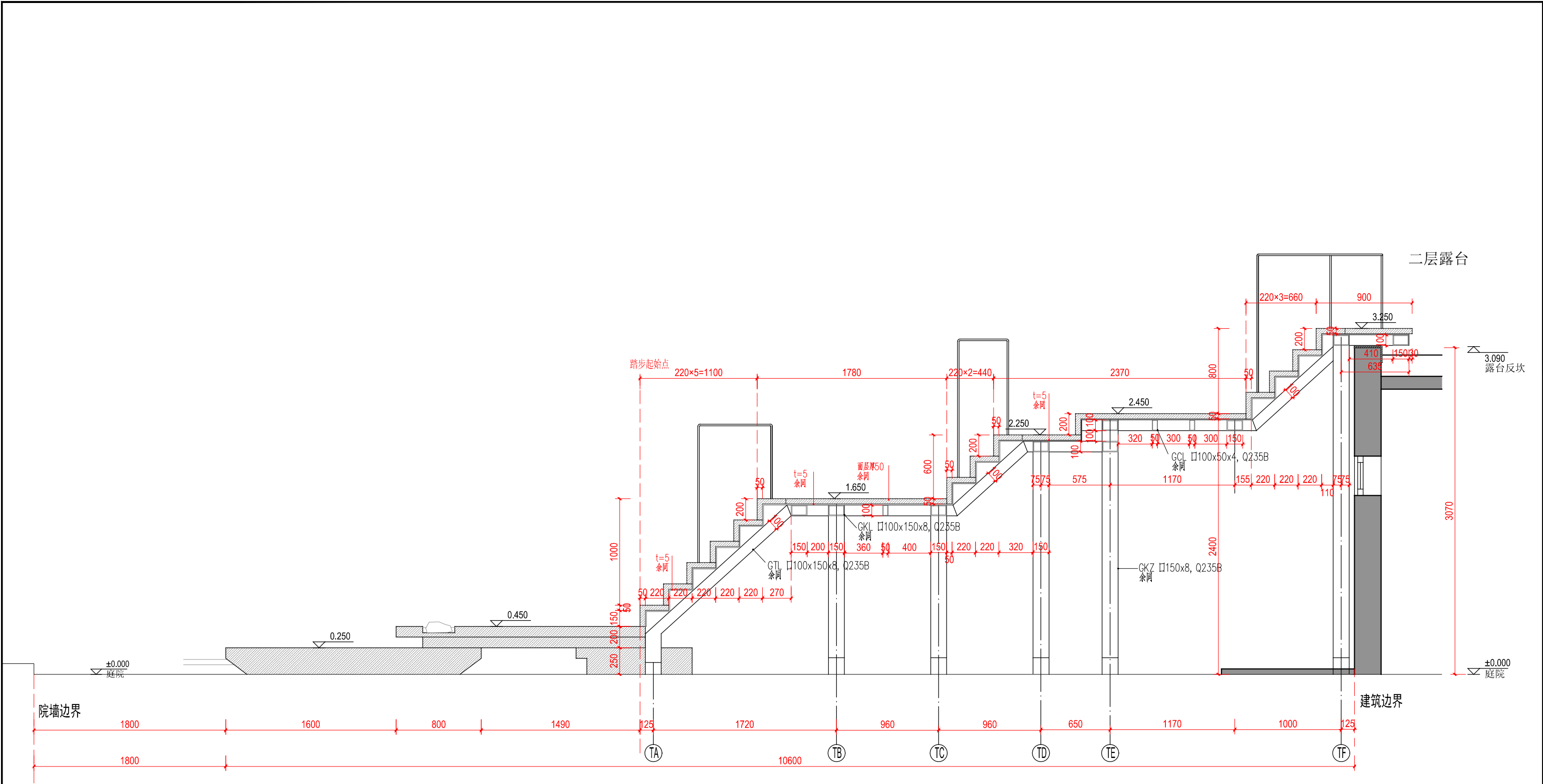
1-1剖面详图
