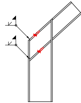
钢梯梁底端节点 1:10
