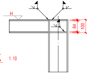
梯梁转折节点 1:10
