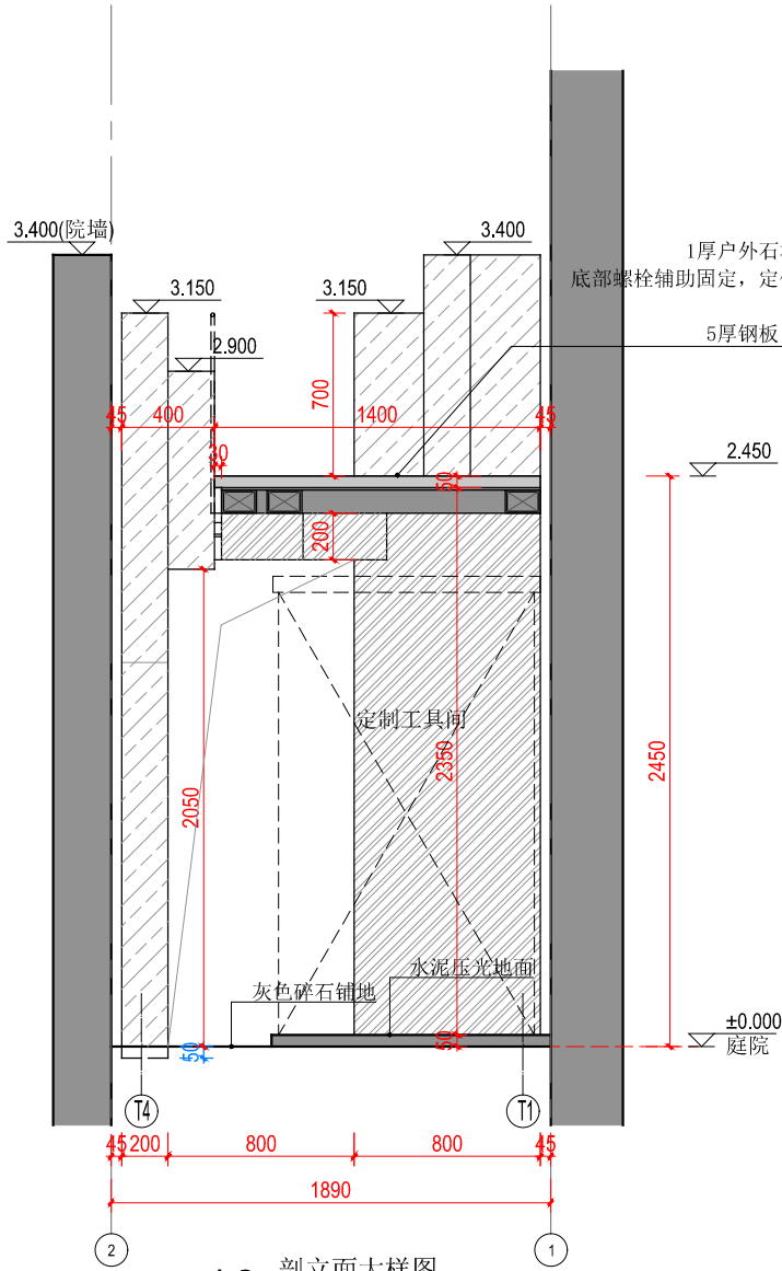
13 剖面大样图 1:20
