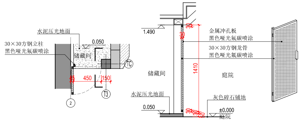
14 剖面大样图 1:20
