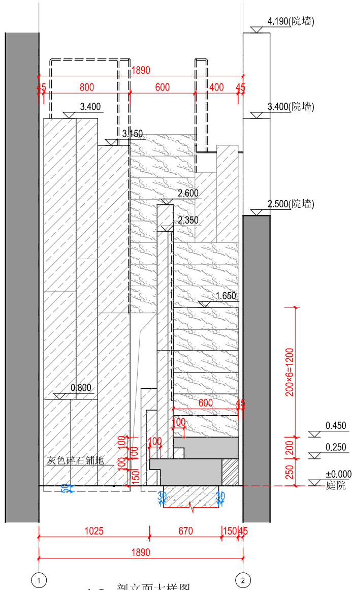
12 剖面大样图 1:20
