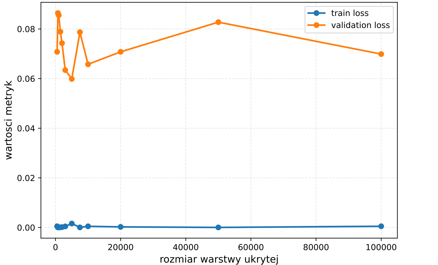
Wpływ rozmiaru warstwy ukrytej na metryki modelu mnist na zbiorze mnist
