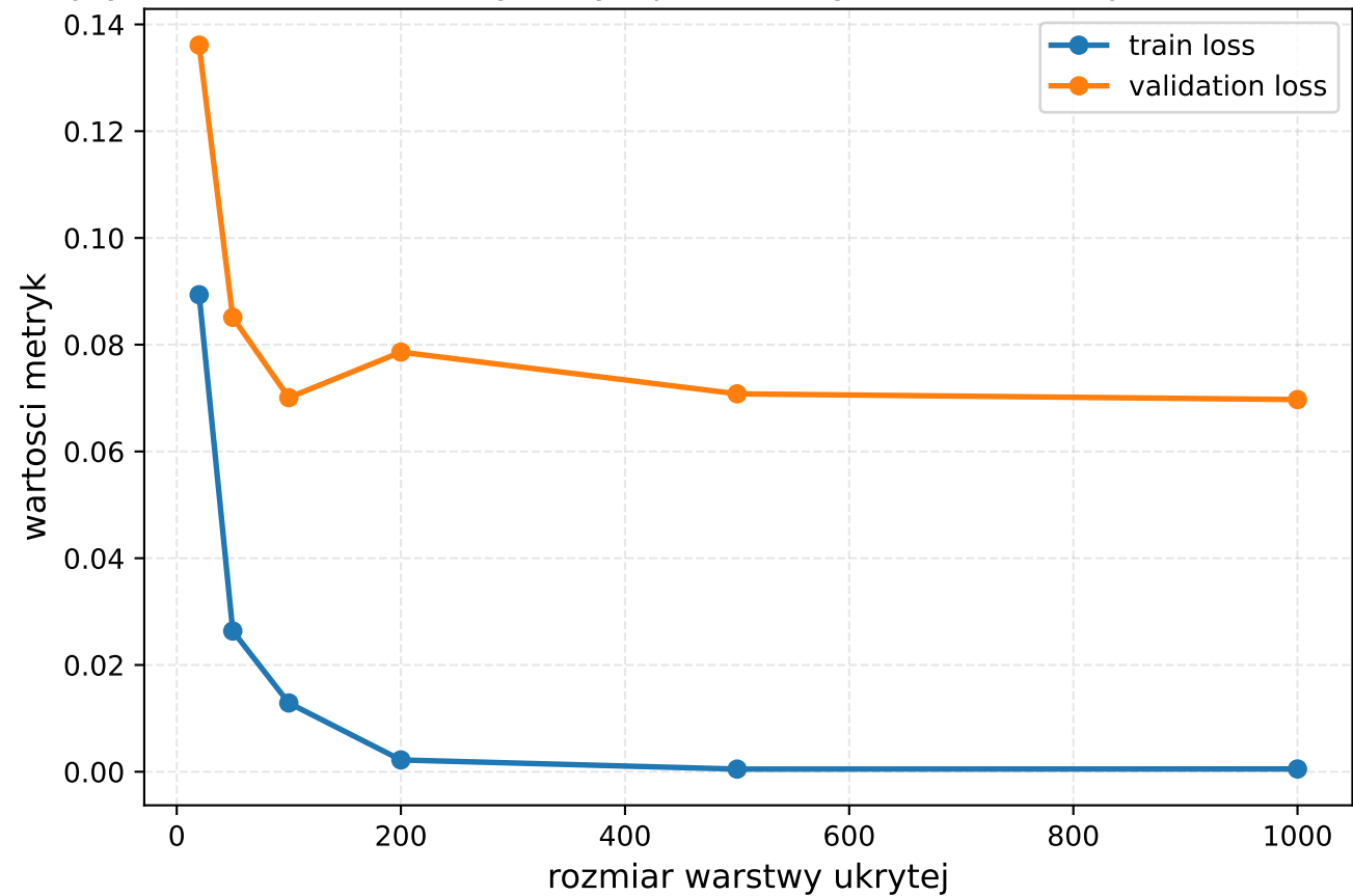
Wpływ rozmiaru warstwy ukrytej na metryki modelu mlp na zbiorze mnist
