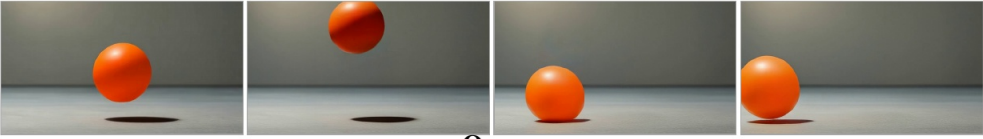
Ours
