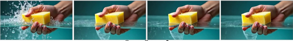
Open-Sora-v2
