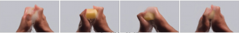
CogVideoX-5B
