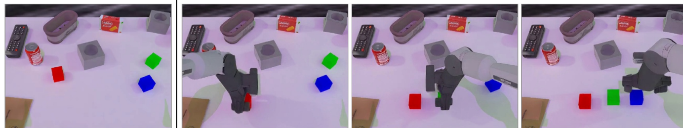
Ours
