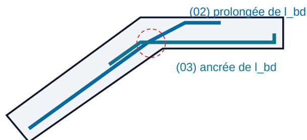
Figure 16 - Angle rentrant : les barres inférieures sont croisées et ancrées de l_{bd} , jamais coudées.
