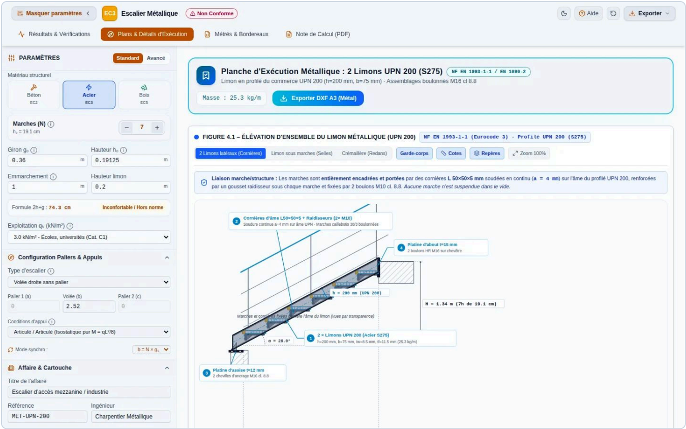
Figure 10 – Élévation d'un escalier à limons latéraux : le limon côté observateur est au premier plan, les marches sont vues par transparence.
