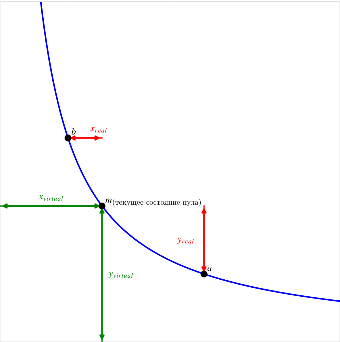
График функции UniswapV3 (CPMM) xy = k
