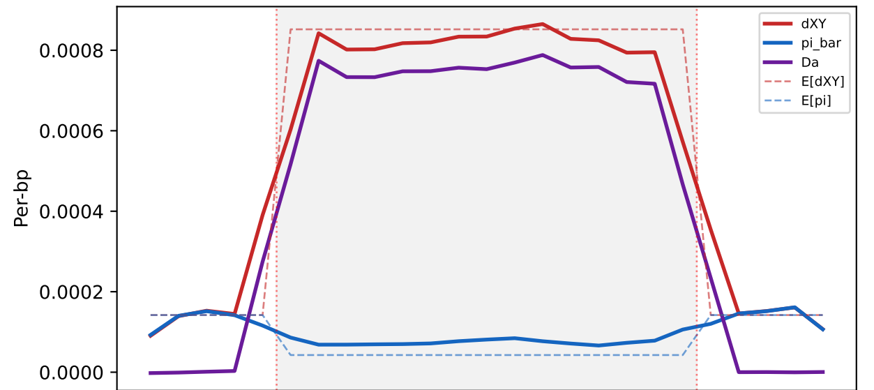
An. funestus 3Ra-like (Ne=10k)
