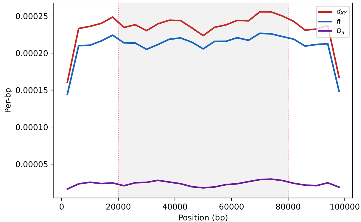
An. funestus 3Ra-like (Ne=44k, t_inv=385k gen)
