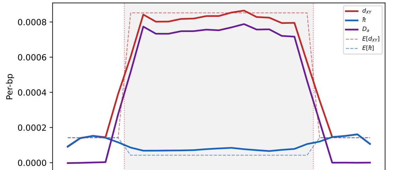
An. funestus 3Ra-like (Ne=10k, t_inv=100k gen)
