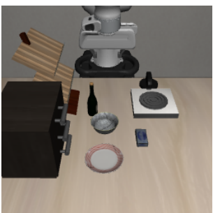
libero_goal/8
