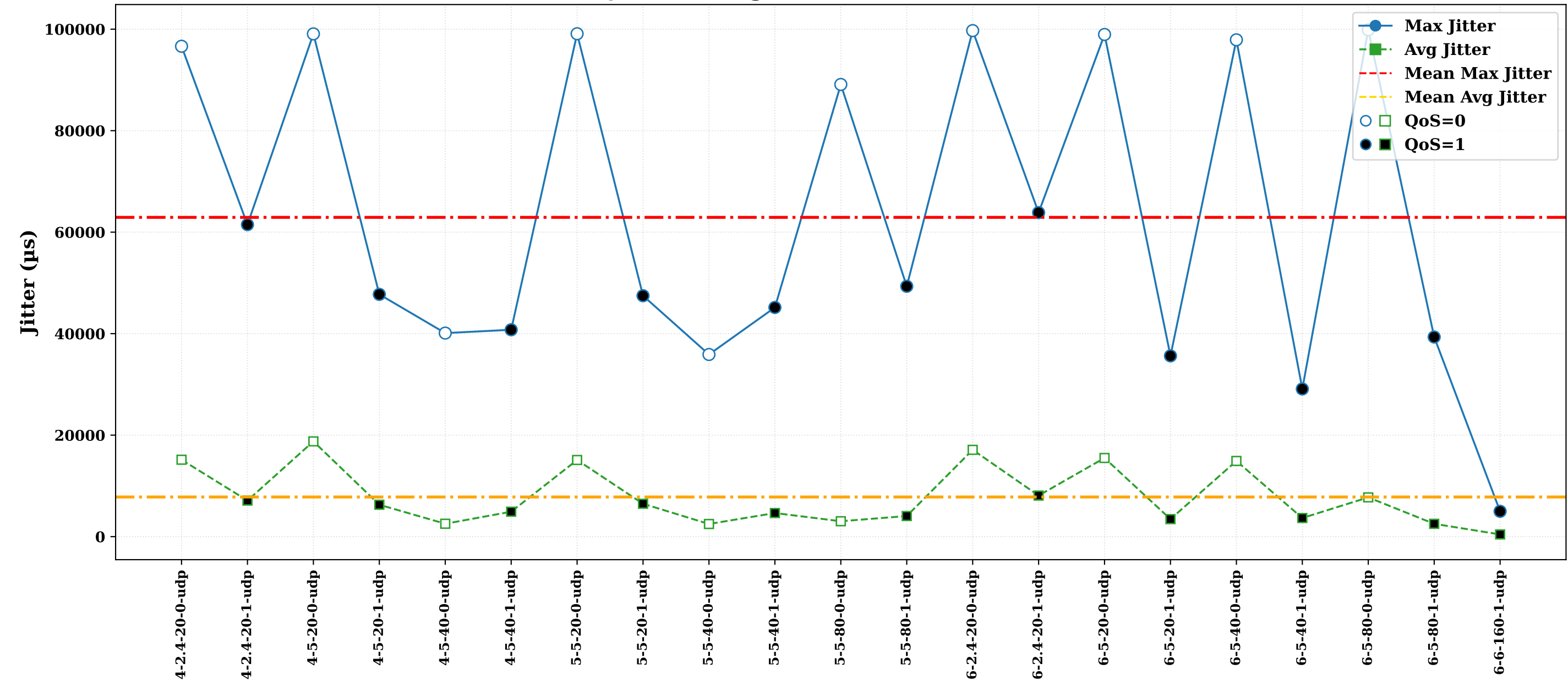
Jitter for high disturbance test (UDP)
