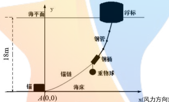
图 1 系泊系统坐标系
