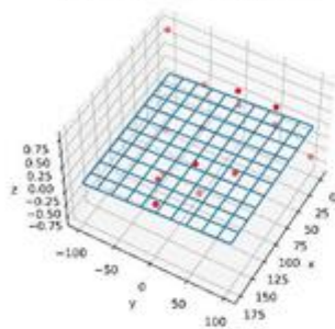
图 27.1 调整前拟合平面
