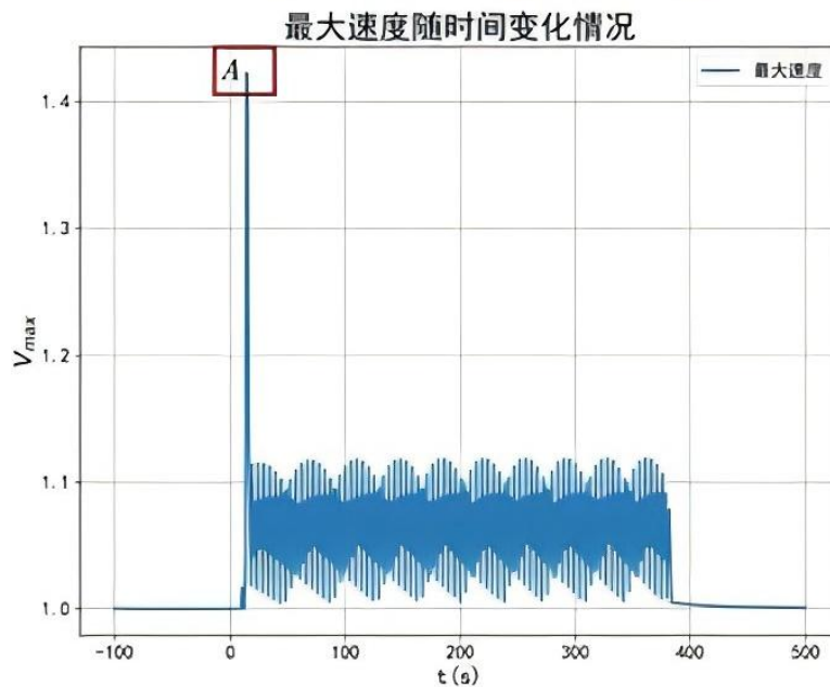
图10 最大速度随时间变化情况
