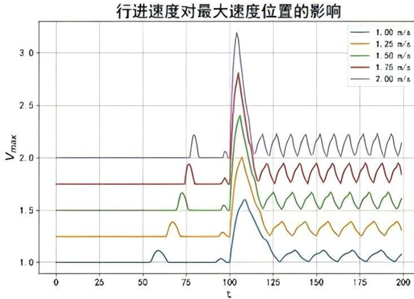
图12 行进速度对最大速度位置的影响
