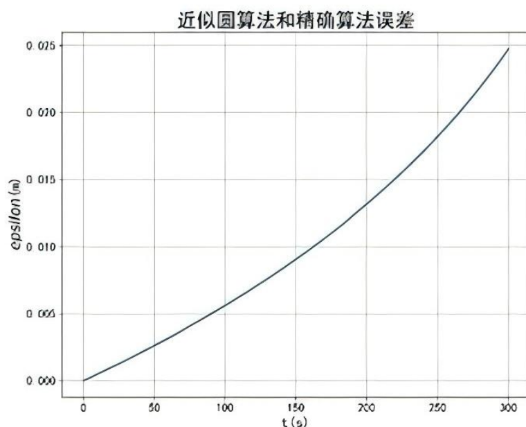
图13 求解结果位置误差
