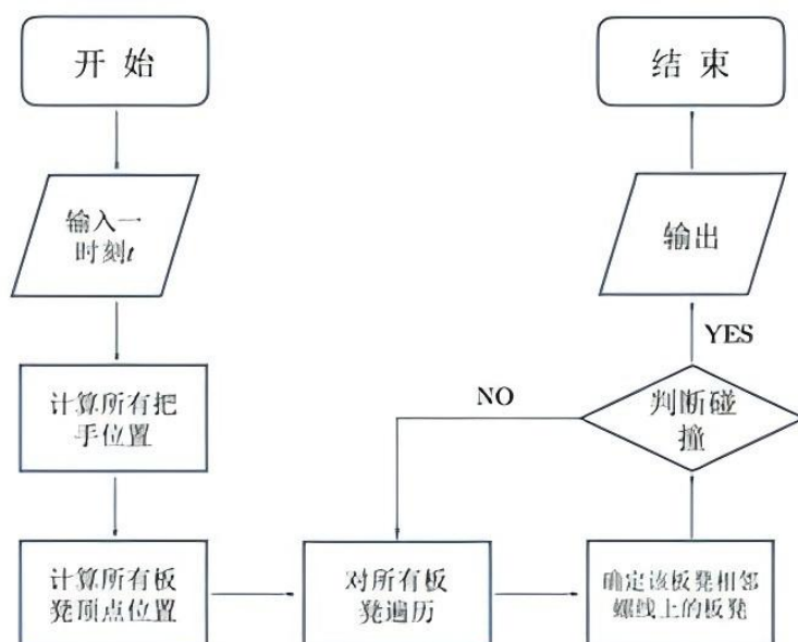
图7 判断碰撞算法流程图
