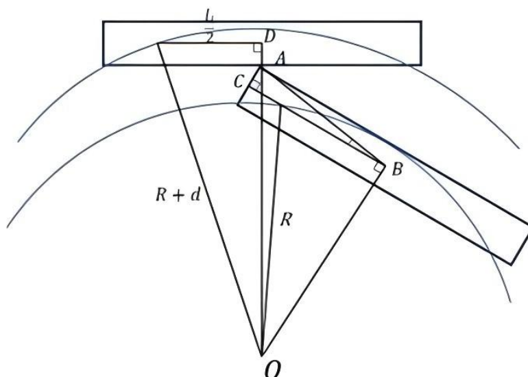
图4 同心圆轨迹碰撞示意图
