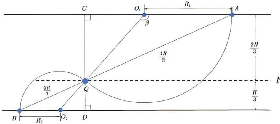
图9 调头空间内几何关系示意图
