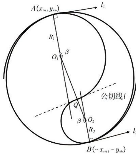
图8 调头空间示意图
